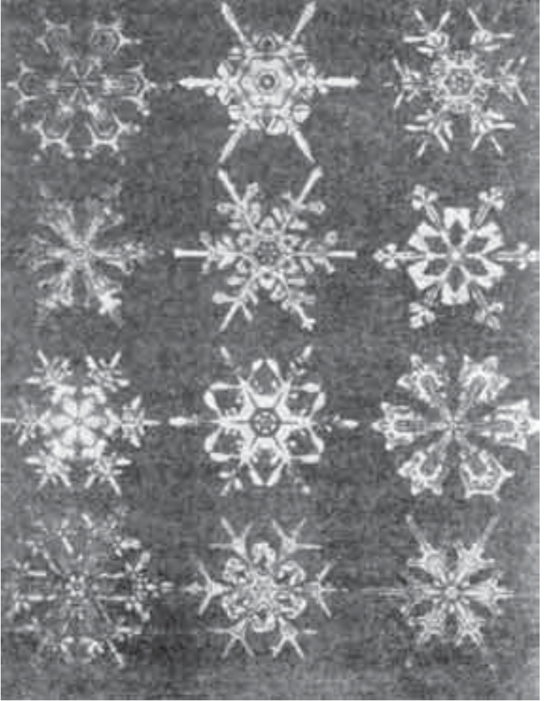
الشكل(3): ندف الثلج
